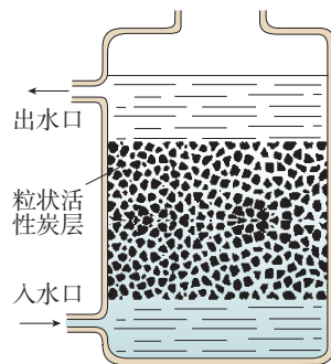
图4-17 活性炭净水器示意图
