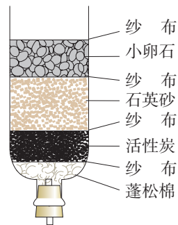
图4-22 简易净水器
