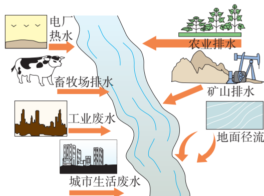
图4-8 水体污染源示意图
