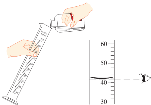
图1-26 液体的量取
