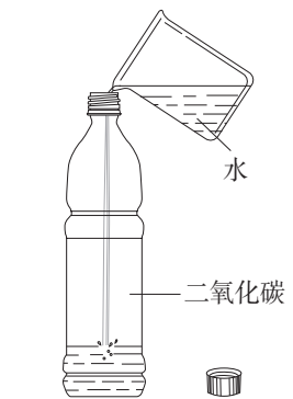
图6-15 二氧化碳的溶解性实验
