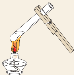
(III) 将通入二氧化碳的试管加热
