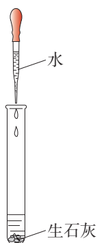
图7-14 生石灰与水反应应放出热量
