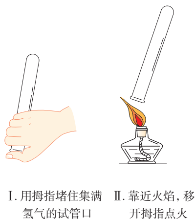
图4-23 检验氢气的纯度
