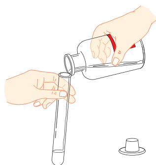
图1-25 液体的倾倒
