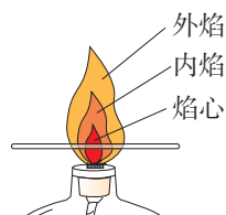
图1-29 酒精灯的灯焰
