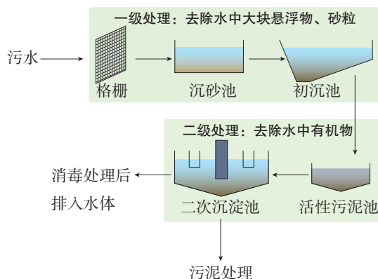
图4-11 污水处理流程示意图
