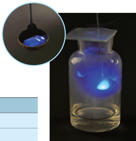
图2-11 硫分别在空气和氧气里燃烧
