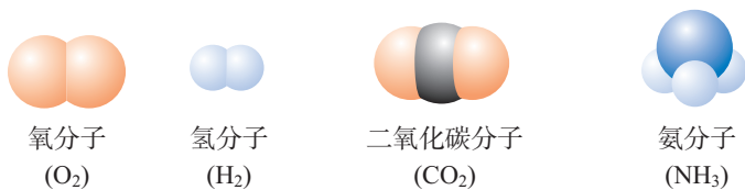
图3-5 几种分子的模型
