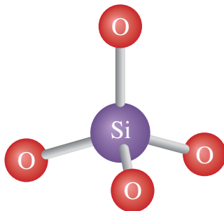
图5-18 硅氧四面体的结构示意图
