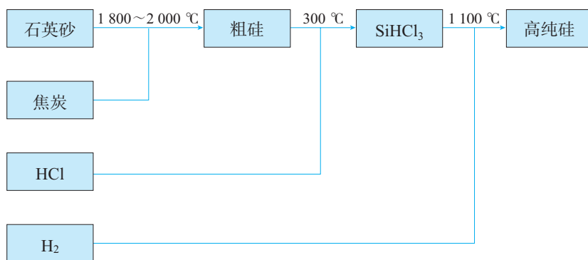
图 5-23 工业制备高纯硅的原理示意图
