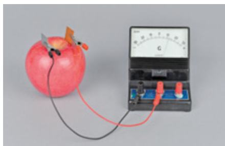
图6-8 水果电池
