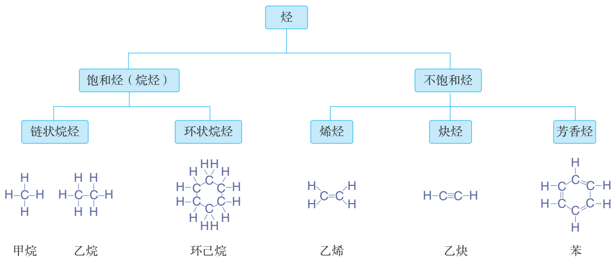
图 7-13 烃的分类
