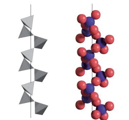
图3-22 石英晶体中的硅氧四面体相连构成的螺旋链
