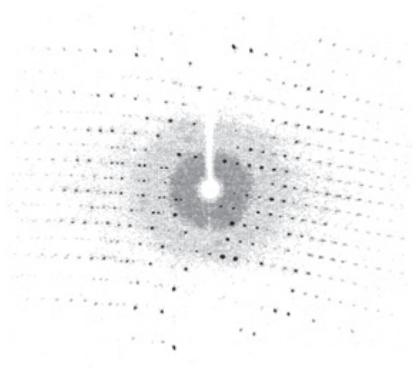
图3-13 单晶衍射图
