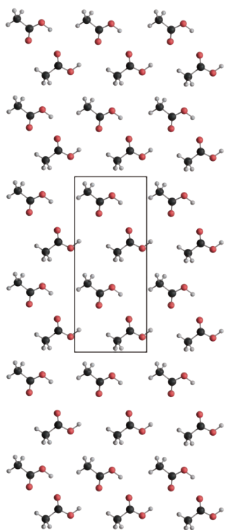
乙酸晶体
