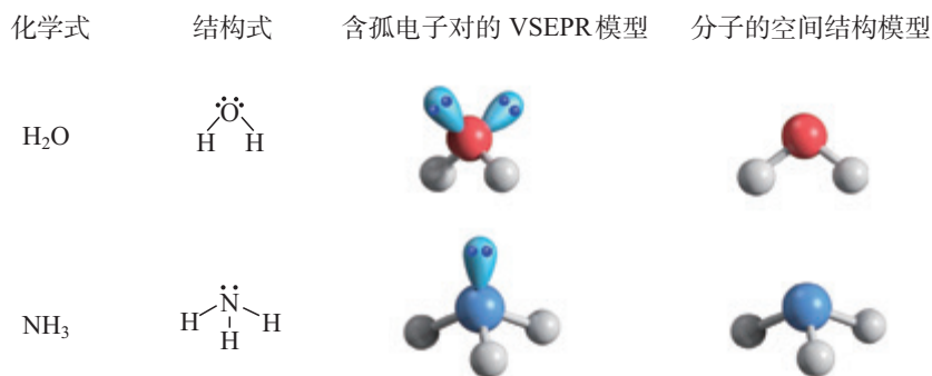
图2-14 \text{H}_2\text{O} 、 \text{NH}_3 的VSEPR模型和空间结构
