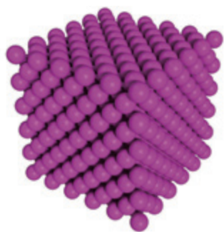
铜晶体
