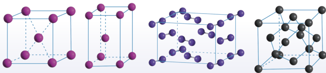
图3-11 钠、锌、碘、金刚石晶胞图
