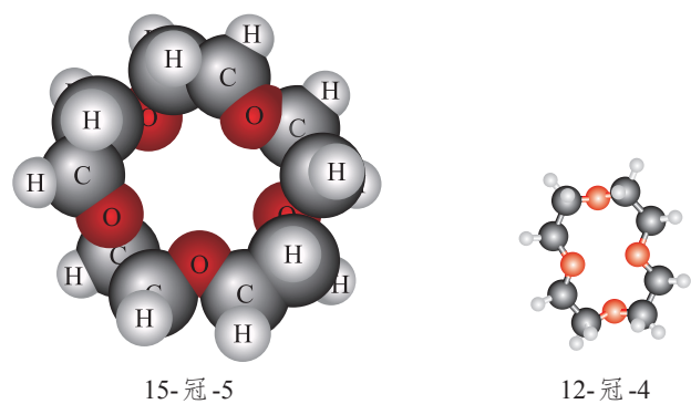
图3-45 冠醚
