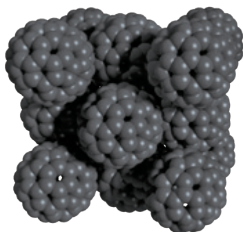
图 3-17 碳 60 的晶胞
