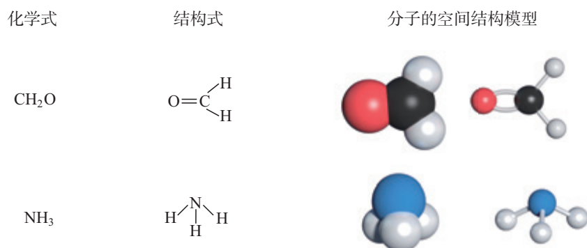
图2-11 \text{CH}_2\text{O} 和 \text{NH}_3 的空间结构模型
