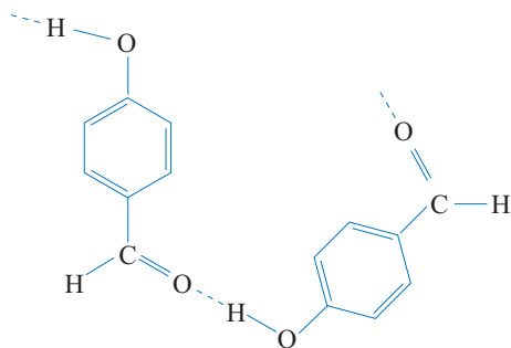
图2-27 分子间氢键
