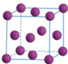
铜晶胞
