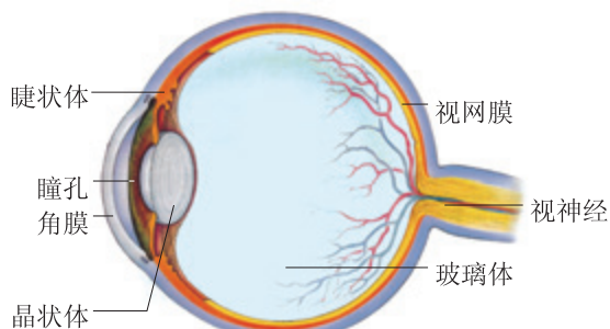
图5.4-1 眼的结构
