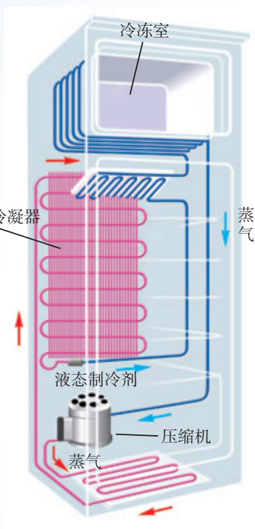
图3.3-8 电冰箱原理图
