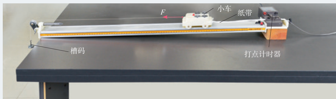
图4.2-2 实验装置
